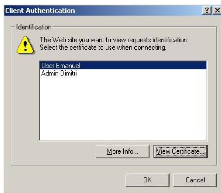
Fig. 1-2. Autentificarea clientului
